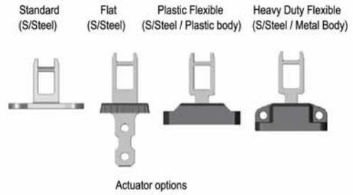
Actuator options
